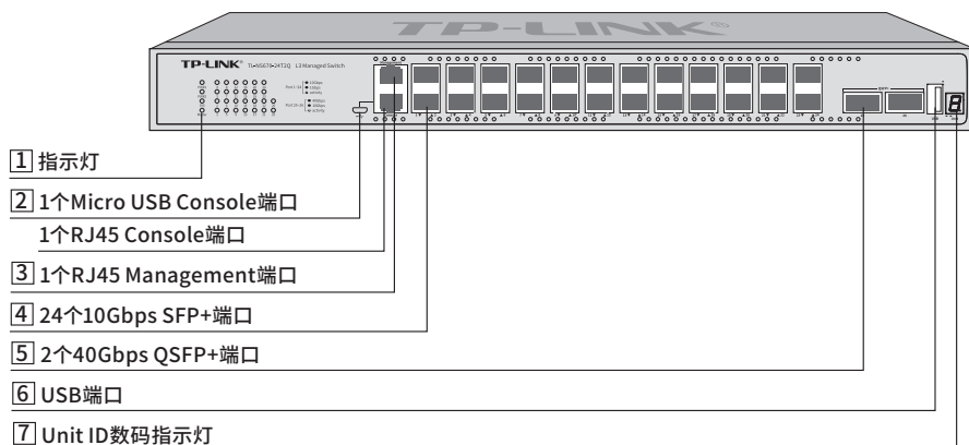
图1-1 TL-NS670-24T2Q前面板示意图
