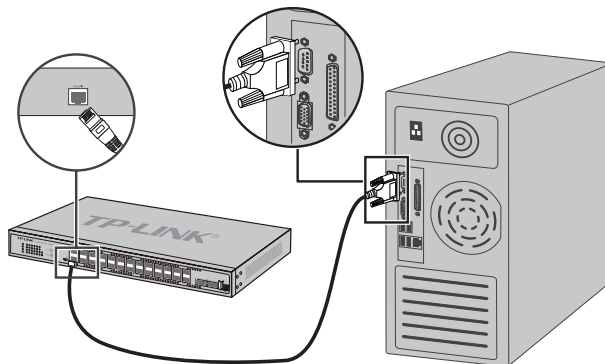
图3-2 RJ45 Console端口连接示意图
