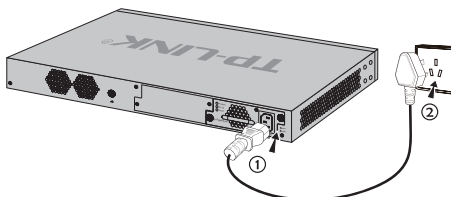
图3-4 电源线连接示意图
