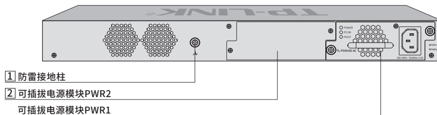
图1-2 TL-NS670-24T2Q后面板示意图
